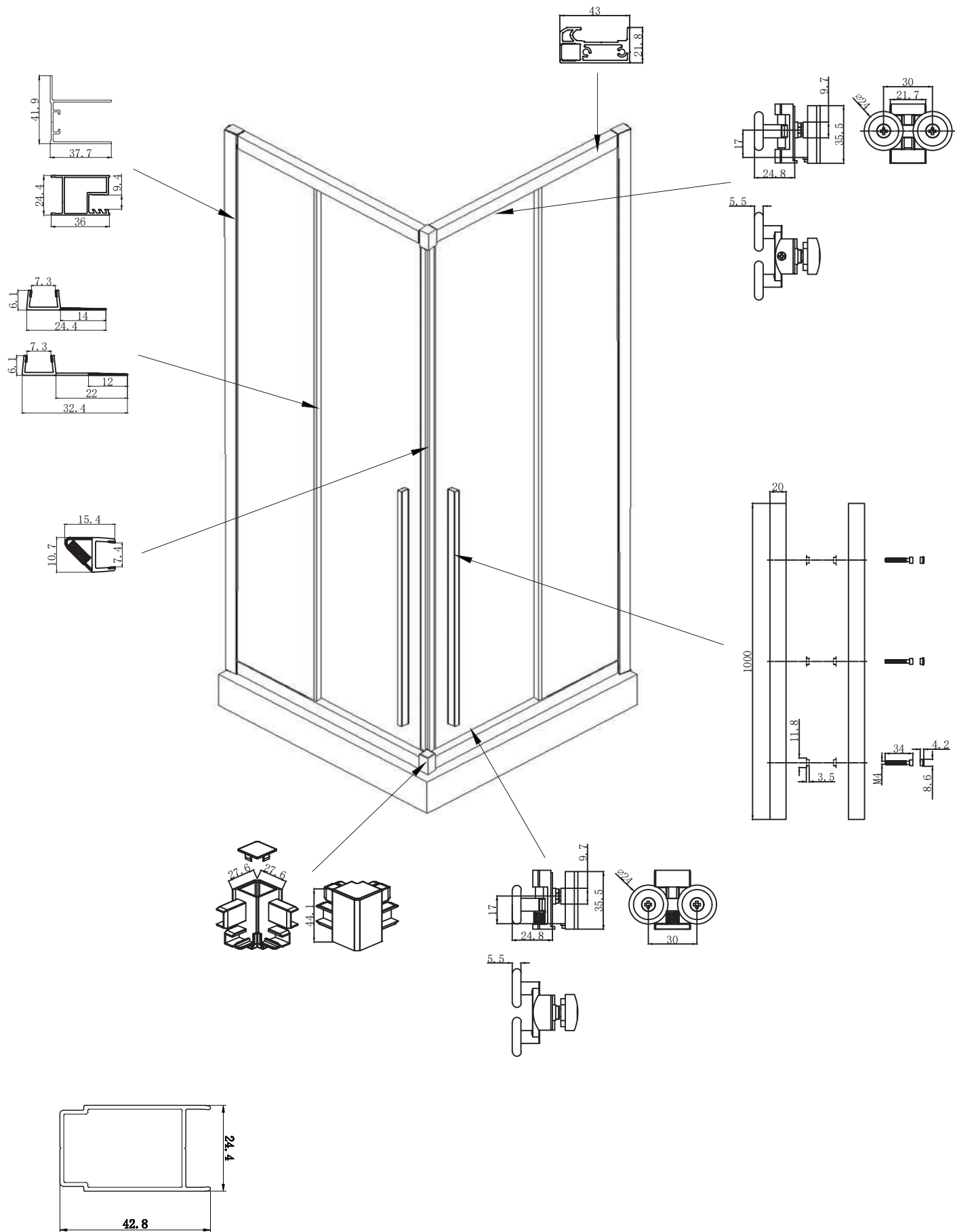
Profilo estensione "11493"
